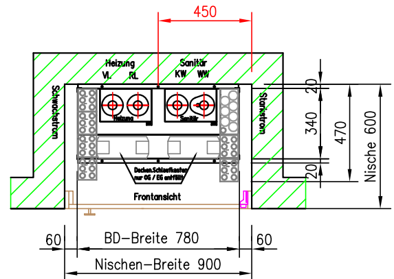
Galip Boden-Durchführung
