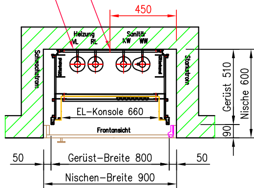
Galip Haustechnik-Gerüst in Mauernische mit bauseitiger Tür-Front
